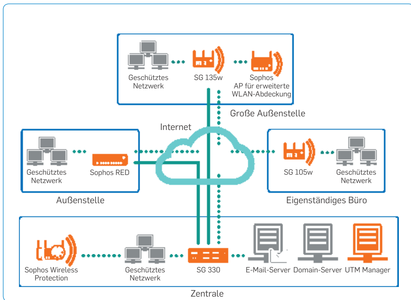
Ein typisches Bereitstellungszenario mit der SG 135w und SG 105w als Teil eines weitverzweigten Unternehmens
